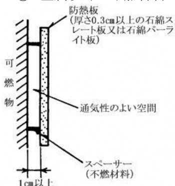
① 金属以外の不燃材料の防熱板
