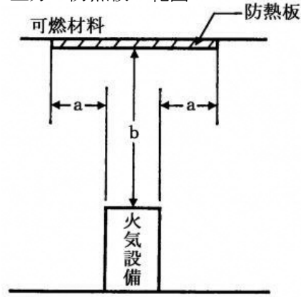
② 上方の防熱板の範囲
