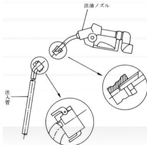
図1 注入管の例
