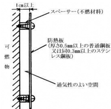
③ ①を金属板で覆ったもの
