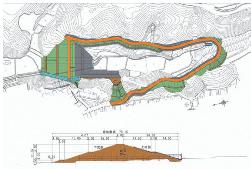
① 西川調節池平面図
