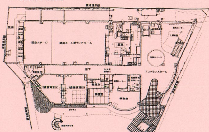
1階平面図
