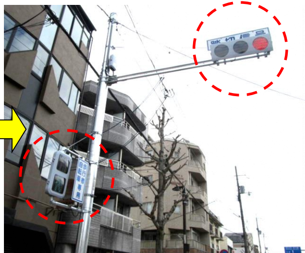
ＬＥＤ式信号機に交換して視認性を改善
