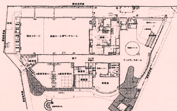
1階平面図
