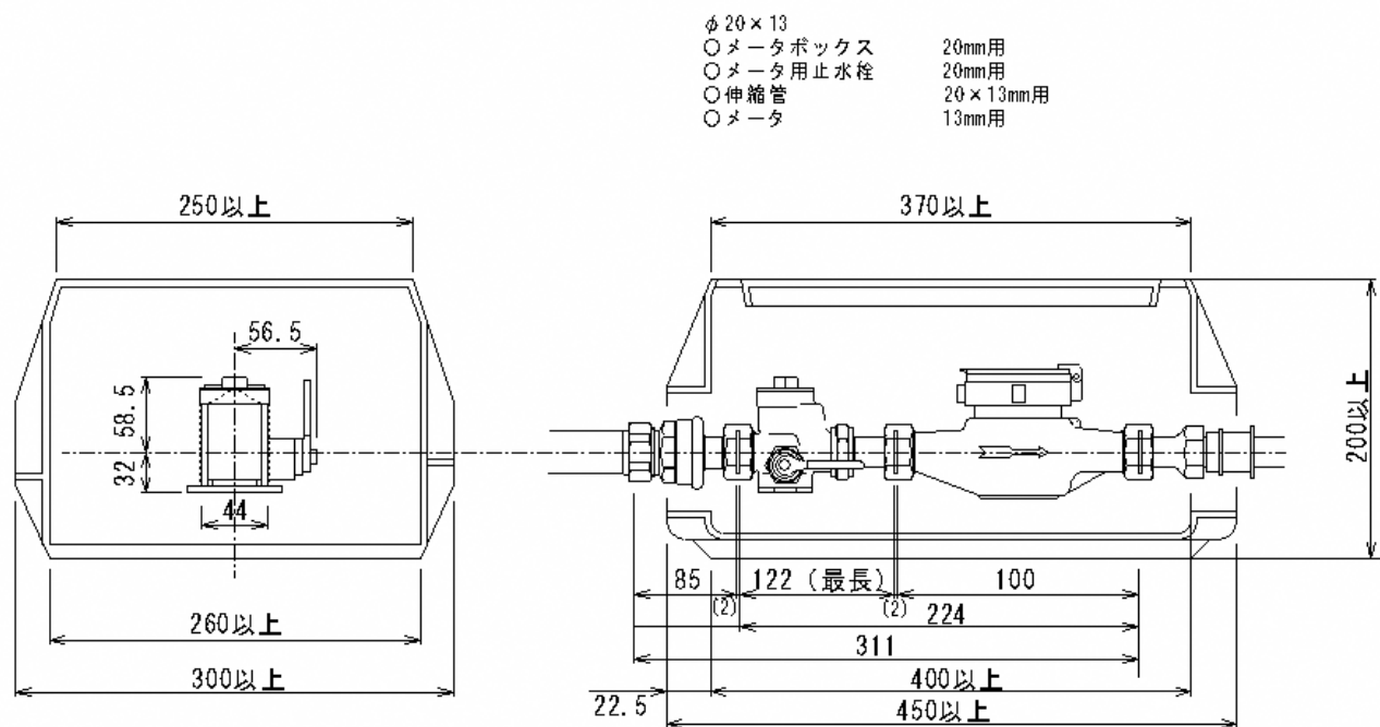
図-3.5.2 \phi 20 \times 13 の場合
