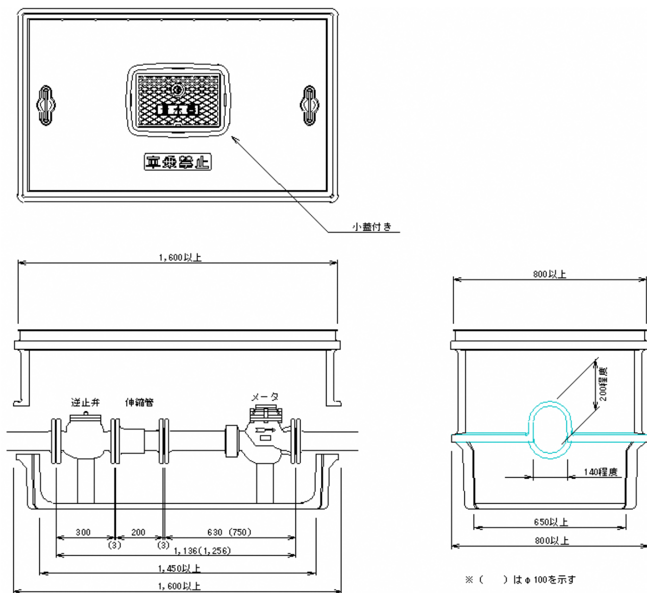
図-3.5.8 \phi 75 、100 の場合
