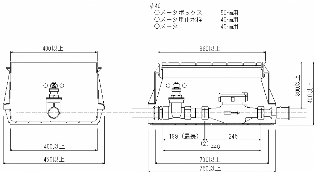
図-3.5.5 \phi 40 の場合
