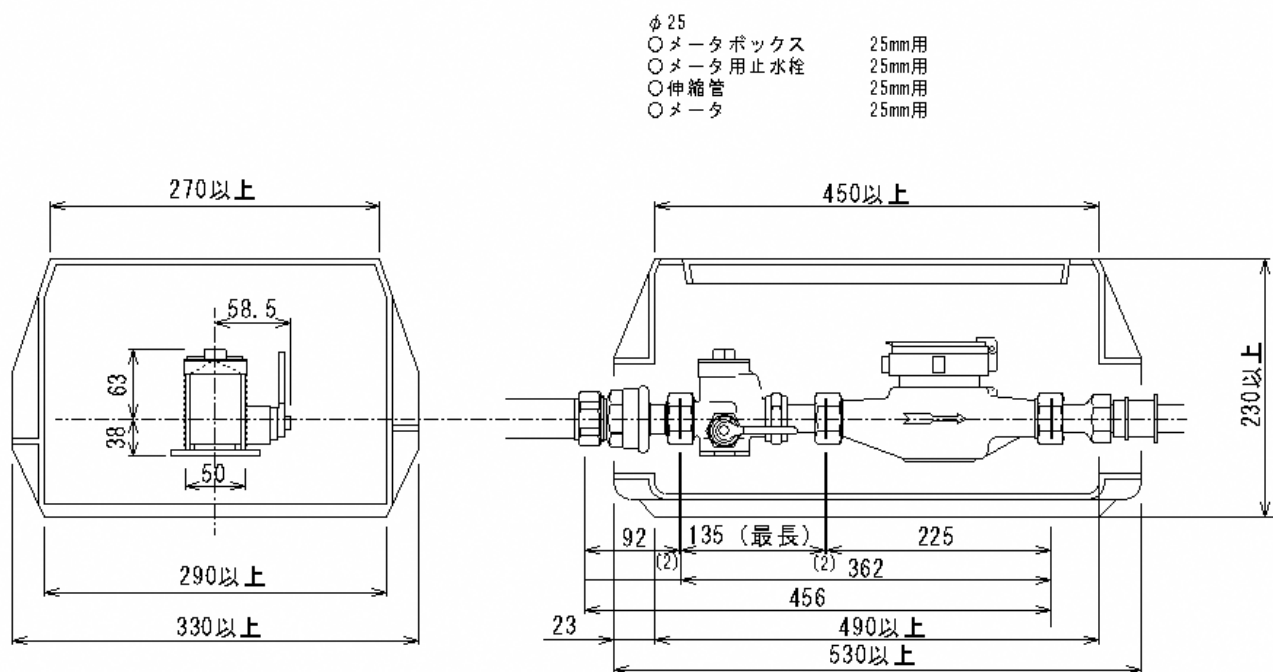
図-3.5.4 \phi 25 の場合
