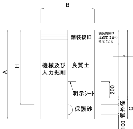
図－3.6.3 給水管布設掘削標準図（ \phi 20 \sim 50 \text{ mm} ）
