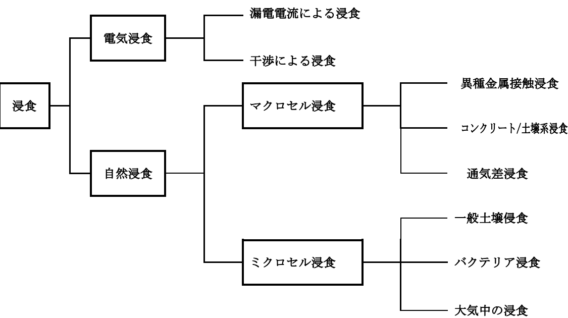
図－3.8.1 金属管の腐食の分類（新版「電気防止対策の手引き」）
