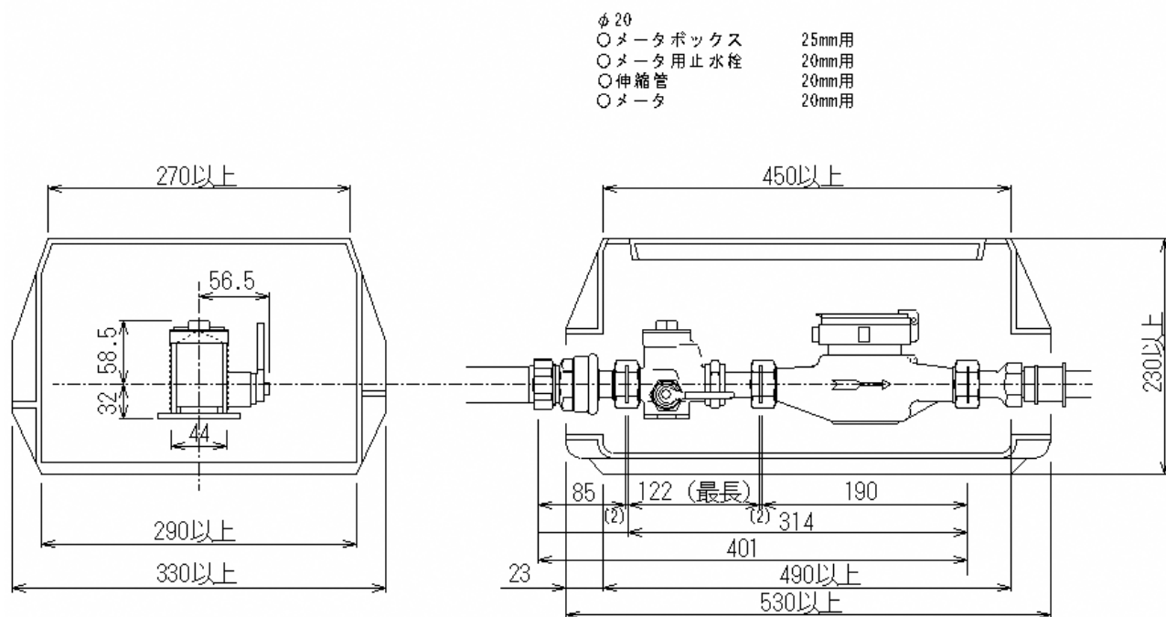
図-3.5.3 \phi 20 の場合
