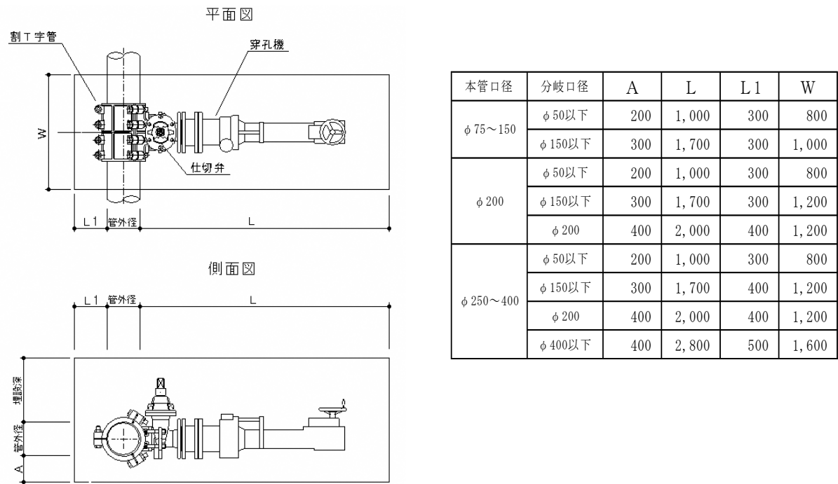
図－3.6.1 割T字管分岐掘削標準図（φ 75～400 mm× φ 50～400 mm）
