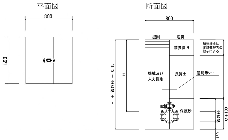
図－3.6.2 分水栓分岐掘削標準図（φ 25～50 mm）
