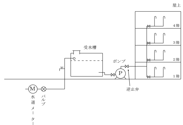
図-2.2.5 ポンプ直送式
