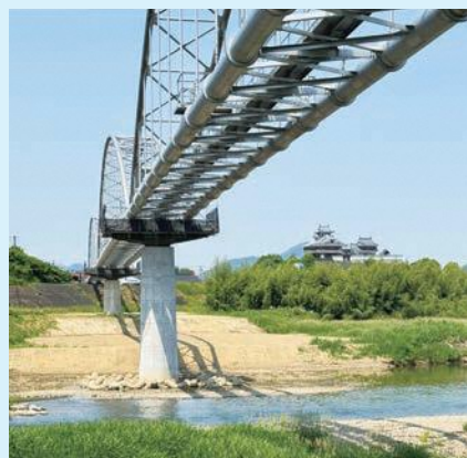
▲土師川水管橋の耐震補強
