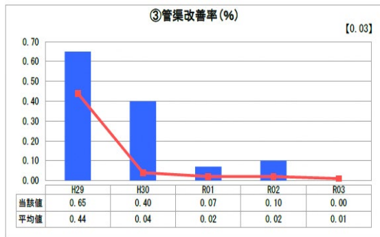
図 1-29 管渠の更新投資・老朽化対策の実施状況
