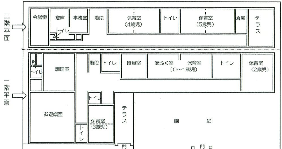
【施設平面図】
