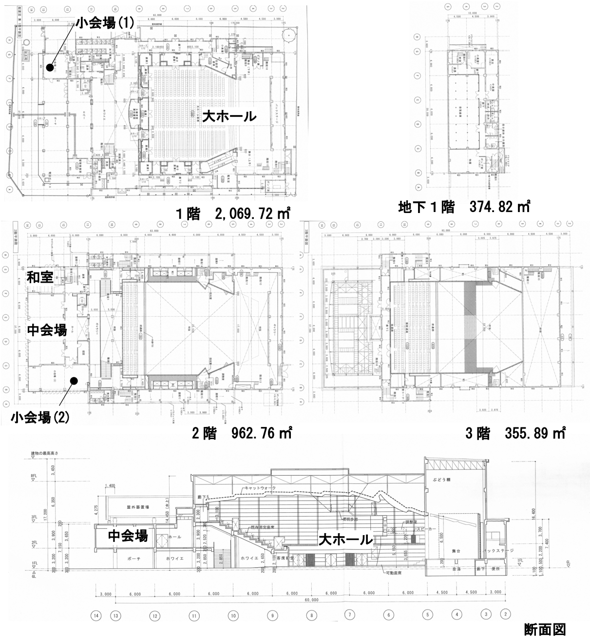
【図 2 施設平面図・断面図】
