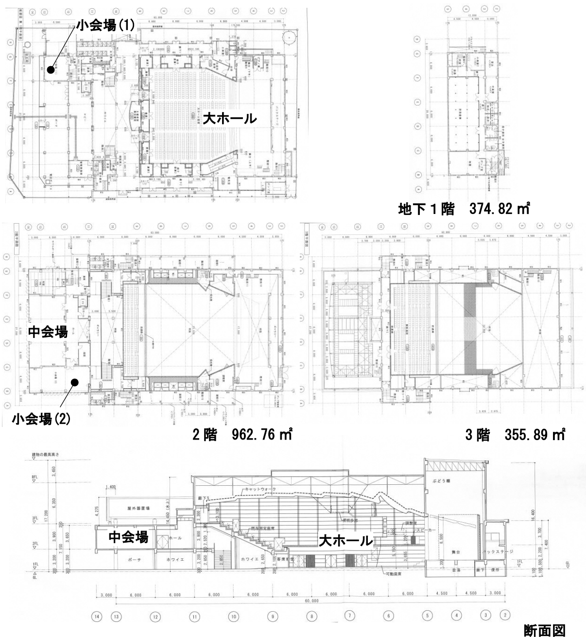
【図 2 施設平面・断面図】
