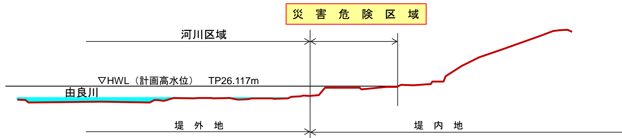
横断面図（42.4km付近）a-a'
