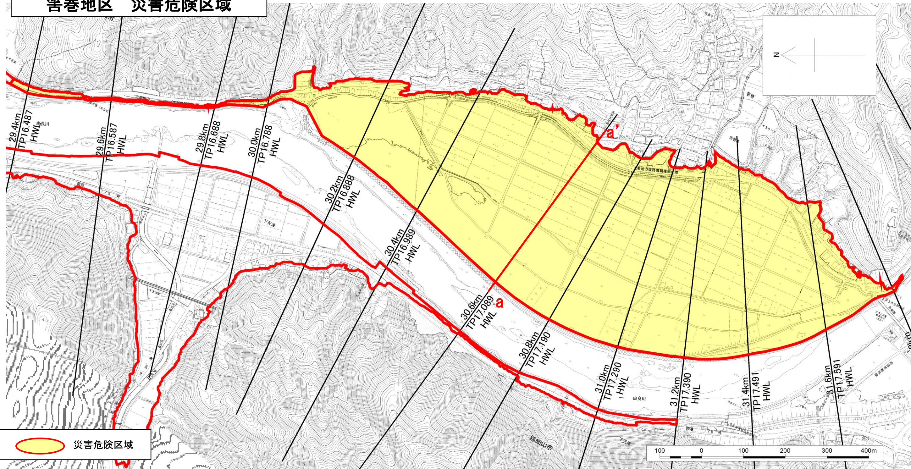
横断図 (30.6km付近) a-a'
