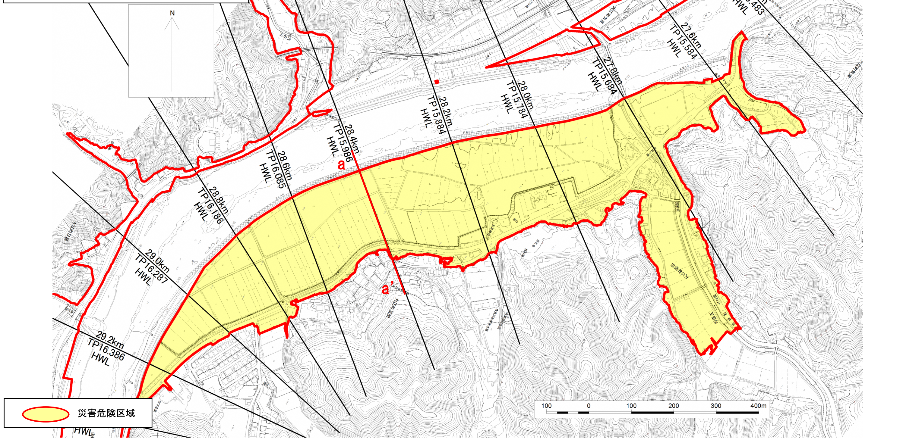
横断図 (28.4km付近) a-a'
