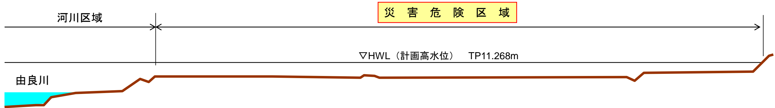
横断図 (19.0km付近) a-a'
