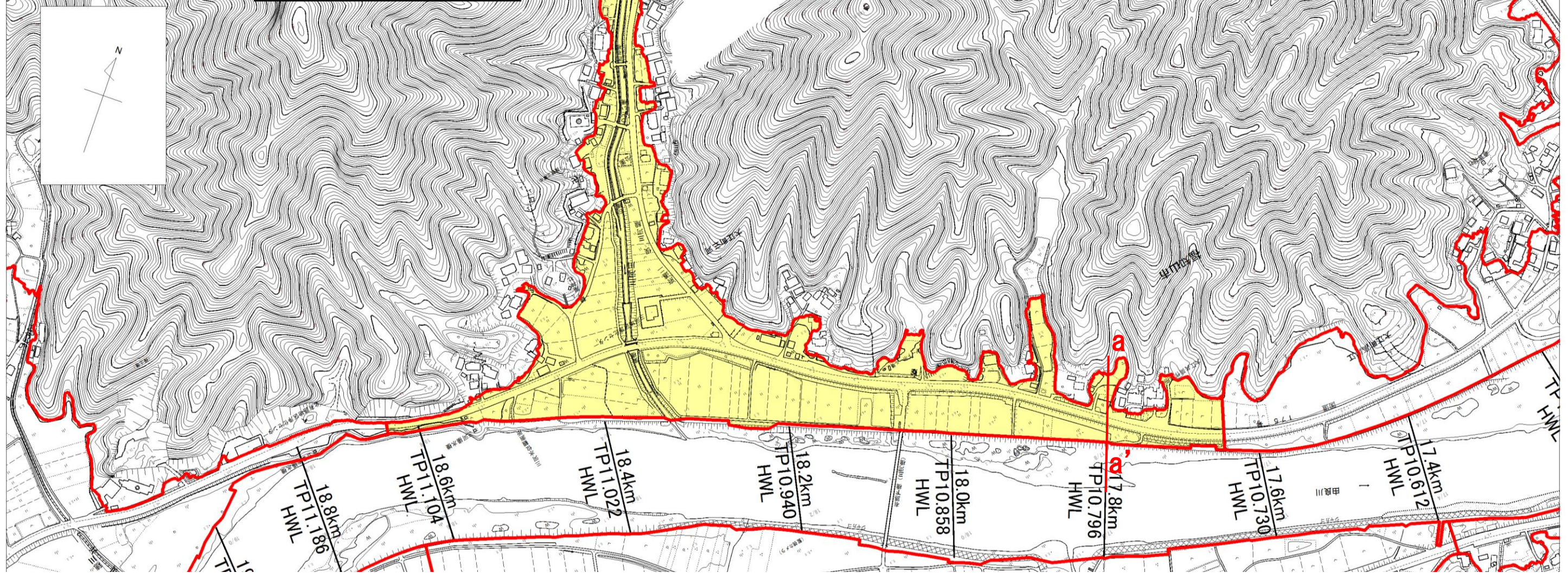
横断図（17.8km付近）a—a'
